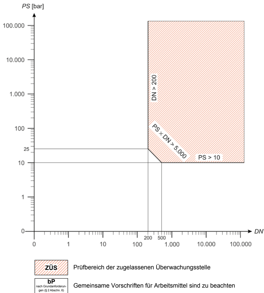
Abbildung 22: Prüfungszuständigkeiten bei Schlauchleitungen nach Nummer 2.2 Satz 1 Buchstabe c für nicht überhitzte Flüssigkeiten, die nach dem Anhang I der Verordnung (EG) Nr. 1272/2008 wie folgt eingestuft werden: als entzündbare Flüssigkeiten in Nummer 2.6 Kategorie 3, wenn die Flüssigkeit höchstens bis zum Flammpunkt erwärmt wird, aber begrenzt auf einen Flammpunkt von 55 Grad Celsius; als ätzend in Nummer 3.2.2.6.
