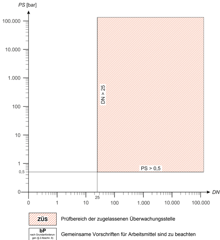
Abbildung 23: Prüfungszuständigkeiten bei Schlauchleitungen nach Nummer 2.2 Satz 1 Buchstabe c für Gase, Dämpfe und überhitzte Flüssigkeiten, die nach dem Anhang I der Verordnung (EG) Nr. 1272/2008 wie folgt eingestuft werden: als entzündbare Gase in Nummer 2.2; als entzündbare Flüssigkeiten in Nummer 2.6 Kategorie 1 oder 2; als entzündbare Flüssigkeiten in Nummer 2.6 Kategorie 3, wenn bei der Verwendung die maximal zulässige Temperatur über dem Flammpunkt liegt, aber begrenzt auf einen Flammpunkt von 55 Grad Celsius; als pyrophore Flüssigkeiten in Nummer 2.9; als akut toxisch in Nummer 3.1.2 Kategorie 1 oder 2.
