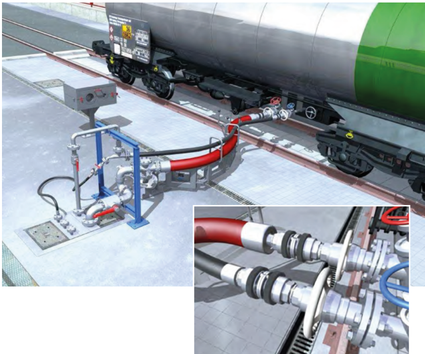
Abbildung 7b: Abreißkupplung mit Wegbegrenzung – Einbaubeispiel
