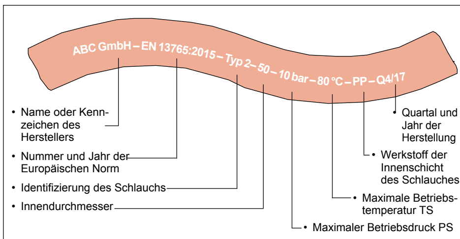
Abbildung 9: Kennzeichnung von Folienwickelschläuchen nach DIN EN 13765 – Beispiel
