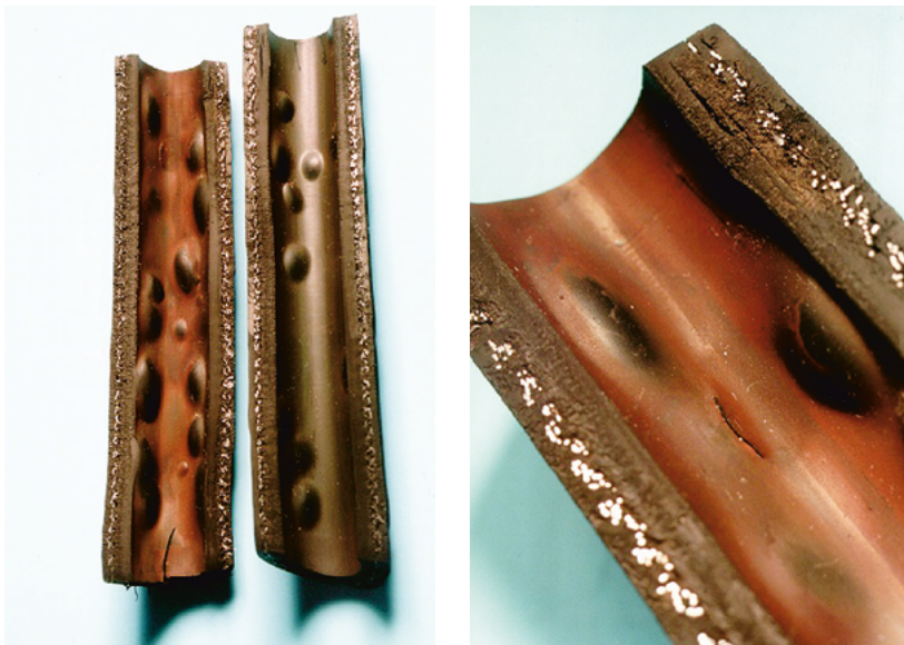
Abbildung 14: „Popcorning“ – Beispiel
