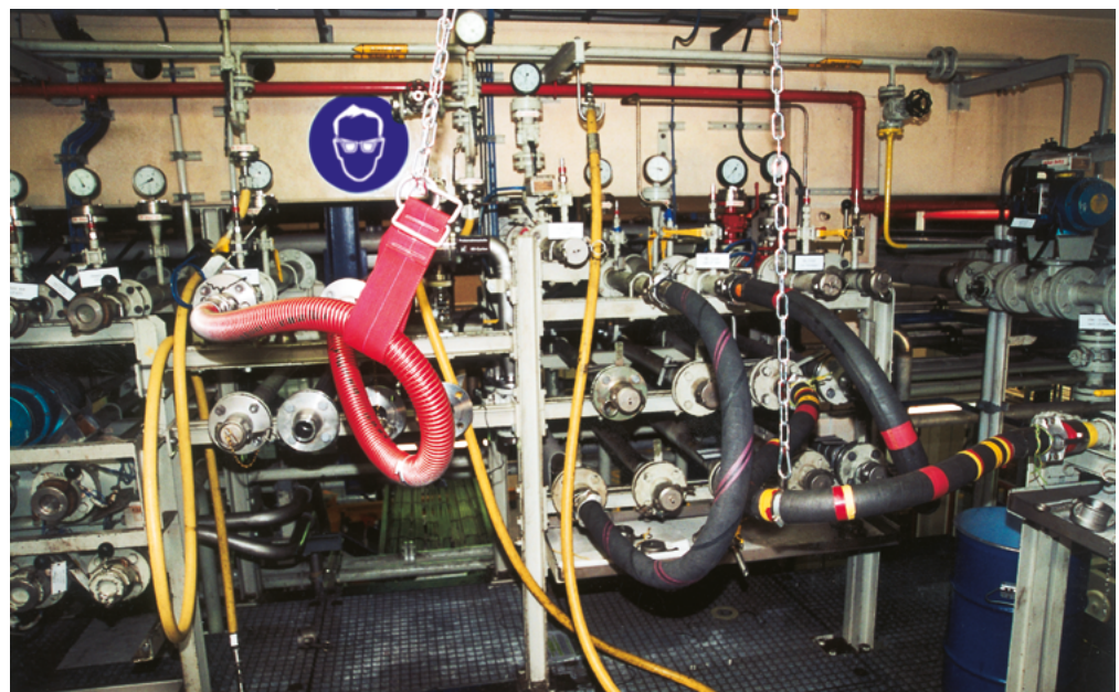
Abbildung 13c: Verlegen von Schlauchleitungen – „Schlauchbahnhof“
