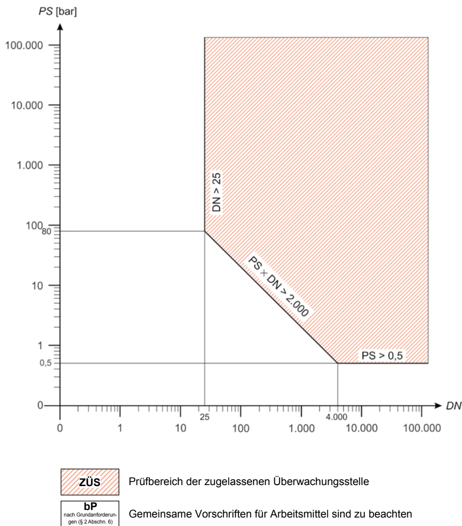
Abbildung 21: Prüfungszuständigkeiten bei Schlauchleitungen nach Nummer 2.2 Satz 1 Buchstabe c für nicht überhitzte Flüssigkeiten, die nach dem Anhang I der Verordnung (EG) Nr. 1272/2008 wie folgt eingestuft werden: als entzündbare Flüssigkeiten in Nummer 2.6 Kategorie 1 oder 2; als entzündbare Flüssigkeiten in Nummer 2.6 Kategorie 3, wenn bei der Verwendung die maximal zulässige Temperatur über dem Flammpunkt liegt, aber begrenzt auf einen Flammpunkt von 55 Grad Celsius; als pyrophore Flüssigkeiten in Nummer 2.9; als akut toxisch in Nummer 3.1.2 Kategorie 1 oder 2.
