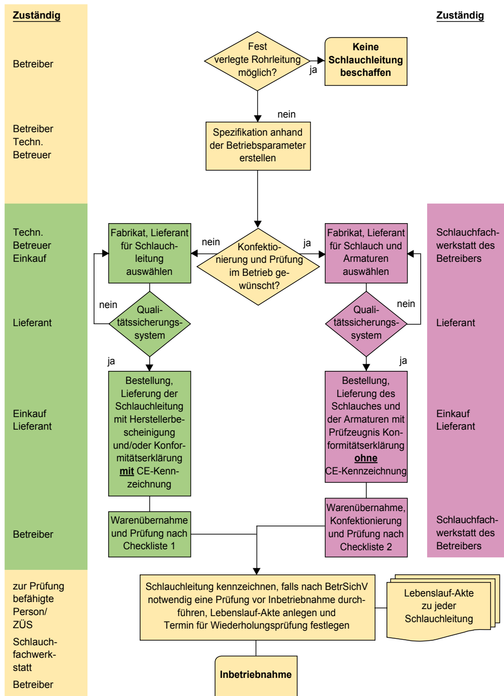
Abbildung 12: Empfehlung für die Beschaffung und Konfektionierung von Schlauchleitungen
